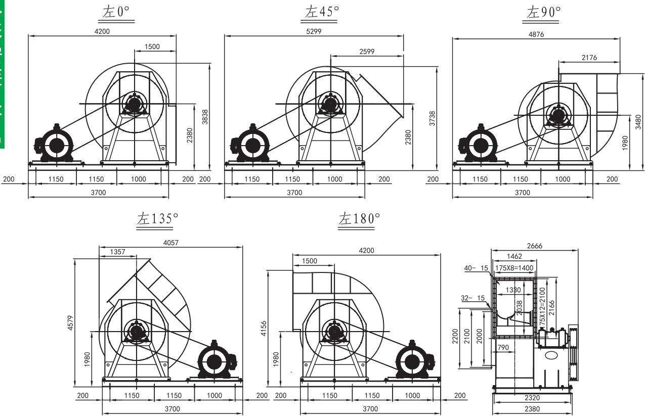
外形安裝尺寸 mm
