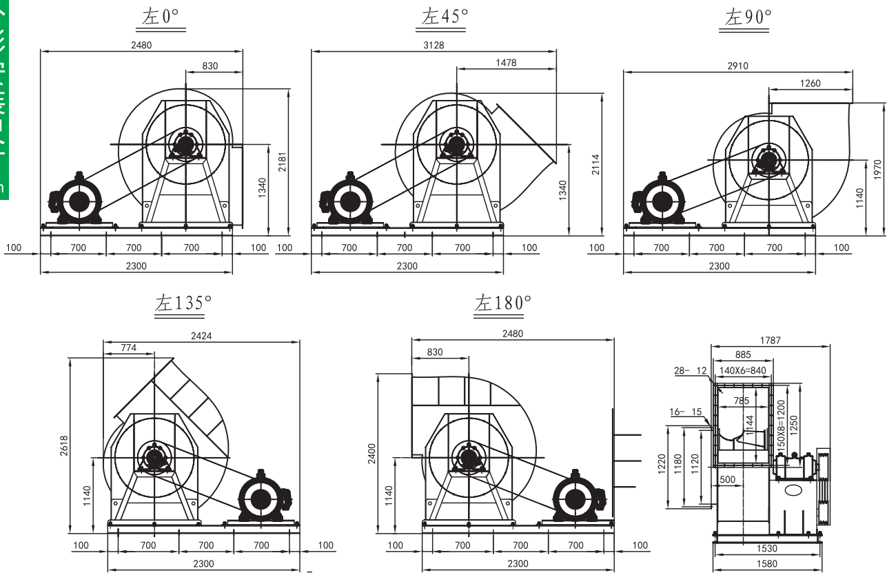
外形安裝尺寸 mm
