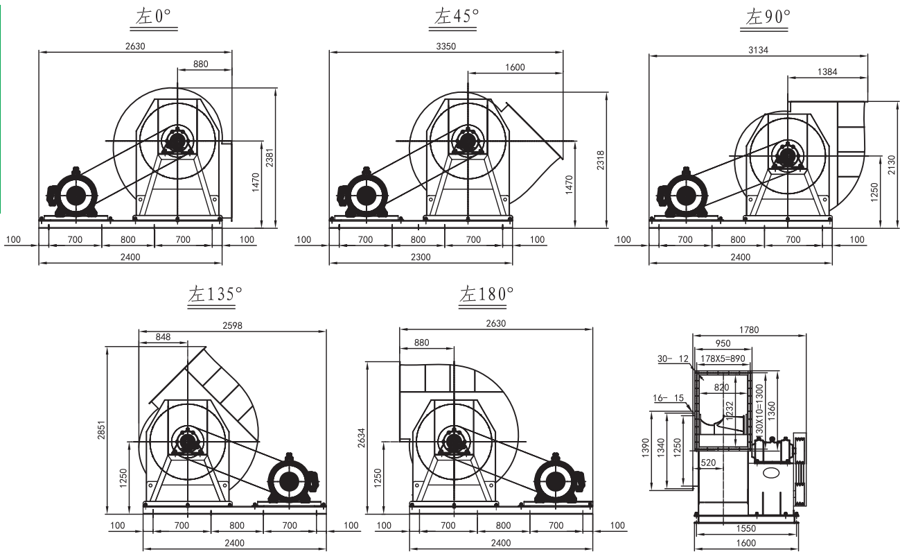
外形安裝尺寸 mm
