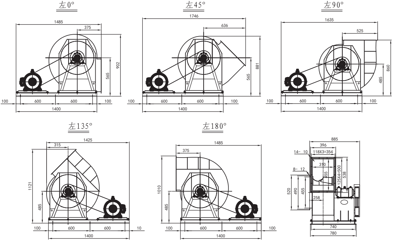
外形安裝尺寸 mm
